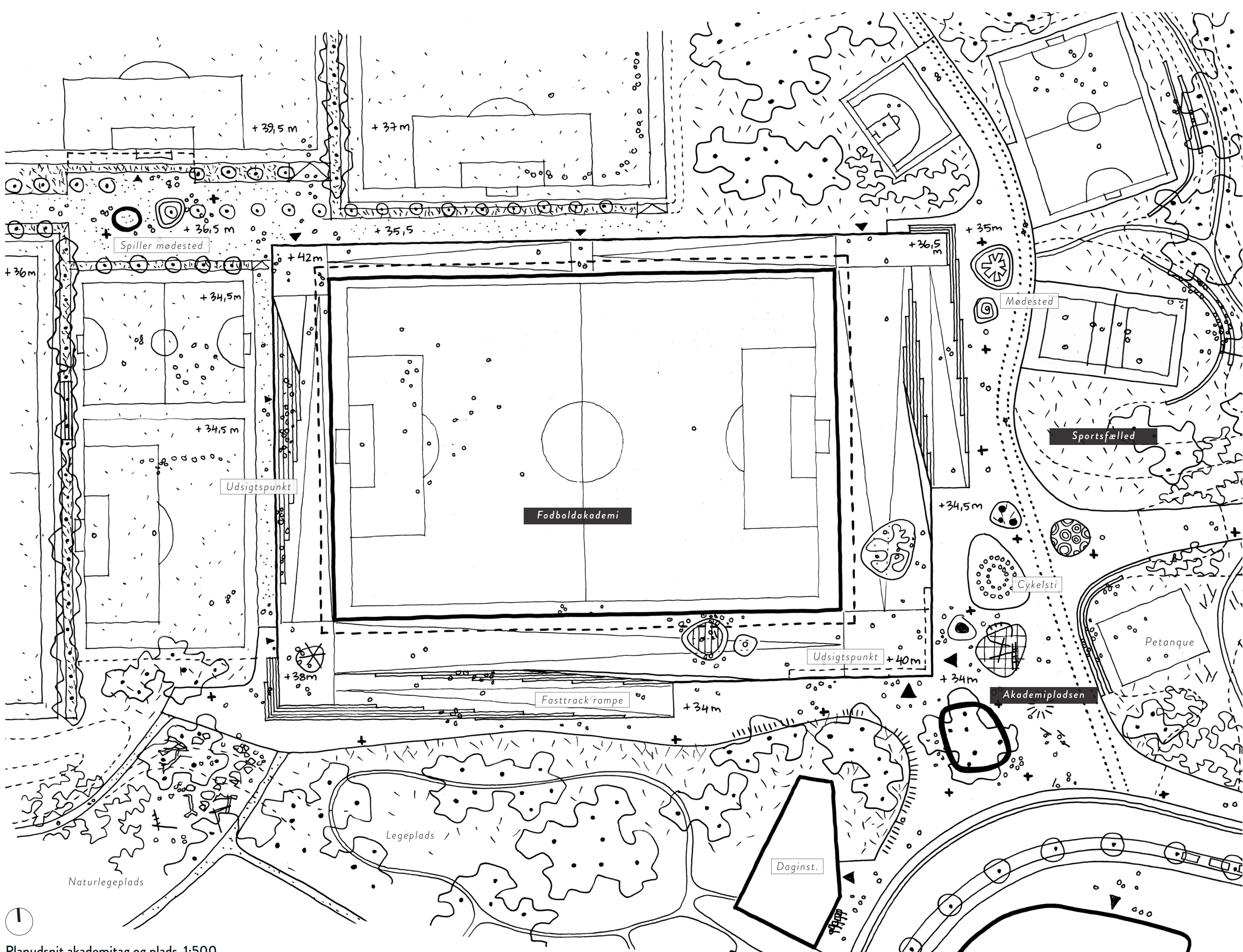
Planudsnit akademitag og plads 1:500
